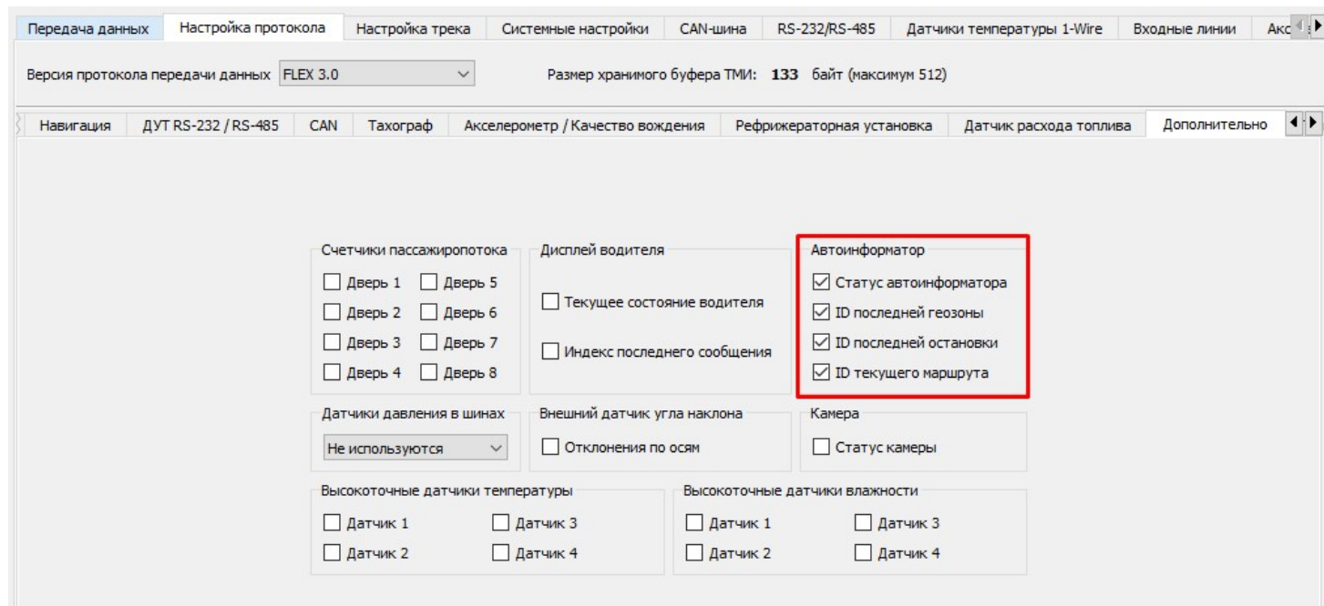
Рис. 133. Настройка протокола для работы с автоинформатором
