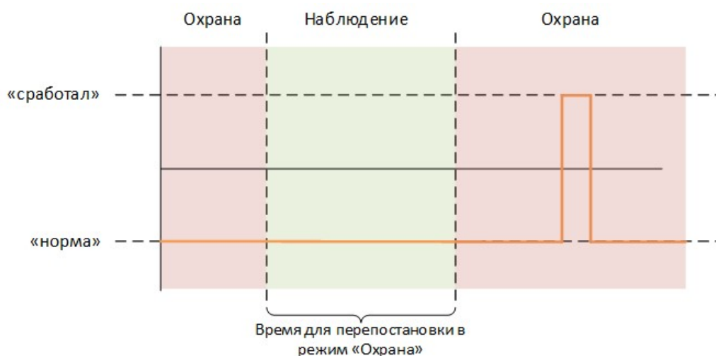
Рис. 148. Пример работы функции «Перепостановка в режим «Охрана»»
