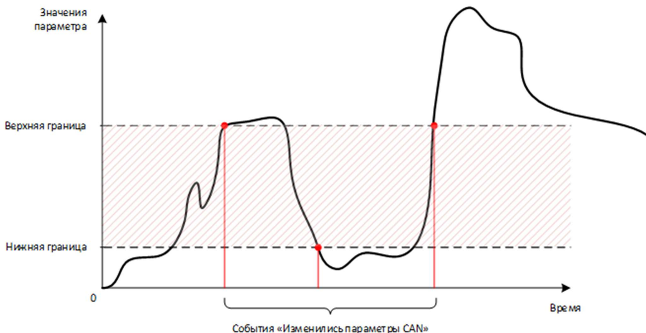
Рис. 78. График, поясняющий работу условия «Переход через границы»
