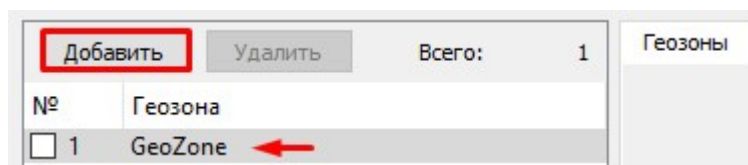
Рис. 118. Добавление геозоны
