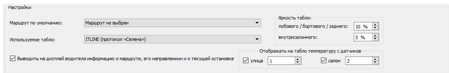
Рис. 123. Настройки автоинформатора
