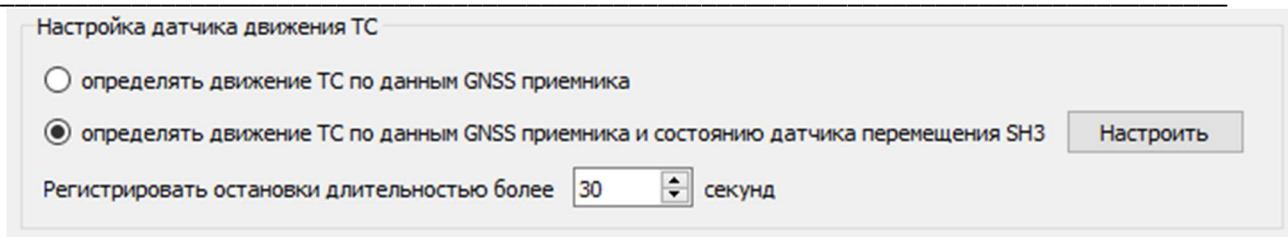
Рис. 38. Настройка датчика движения ТС
