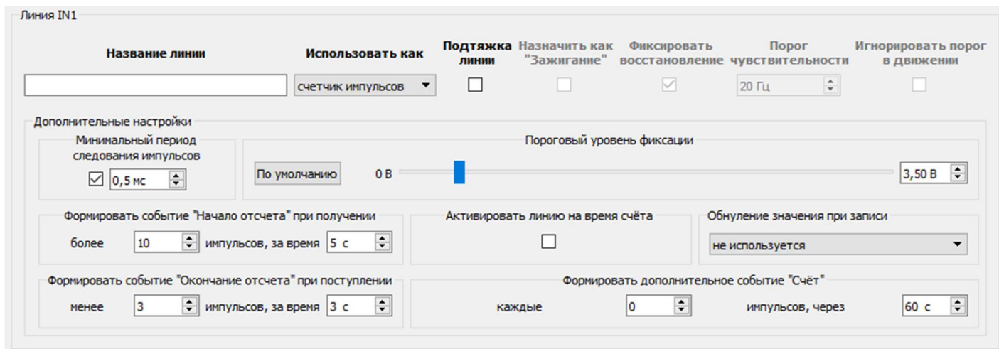
Рис. 95. Настройка входа, как «счетчик импульсов»
