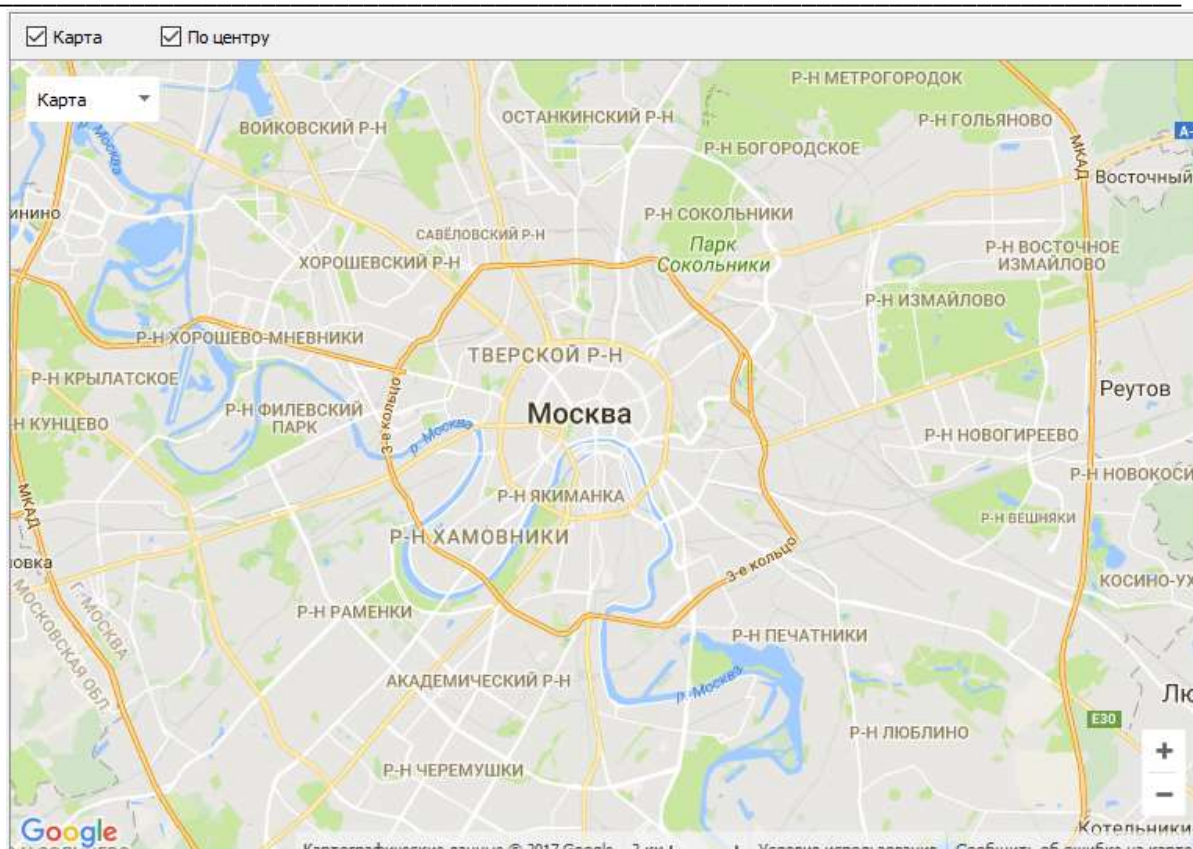
Рис. 117. Окно карты
