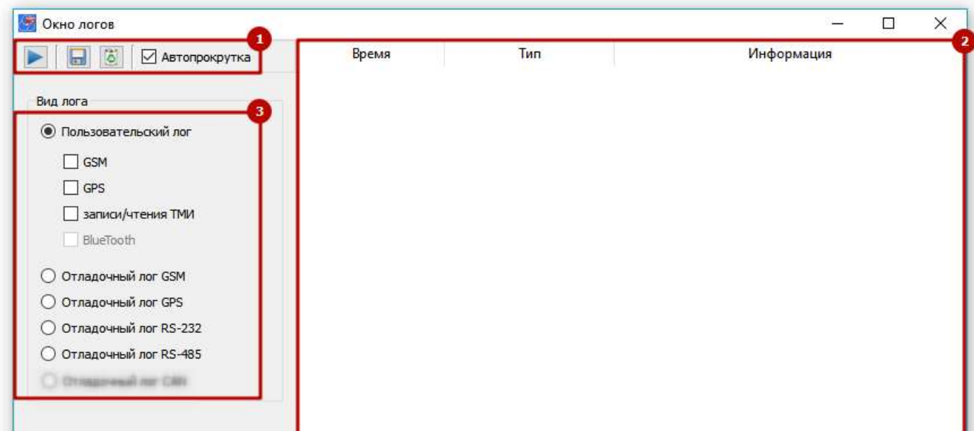
Рис. 16. Окно логов
