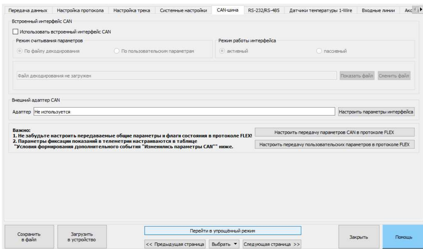
Рис. 59. Вкладка «CAN-шина»
