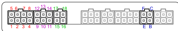
Рис.3. Интерфейсные разъемы дисплея «АвтоГРАФ-ИНФО» (5" TFT / microSD / ГС / ГЛОНАСС+GPS) / (5" TFT / microSD / ГС).
