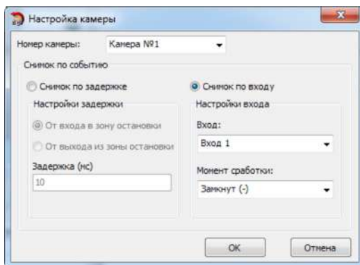
Рис.67. Настройка камеры для съемки на остановках.
