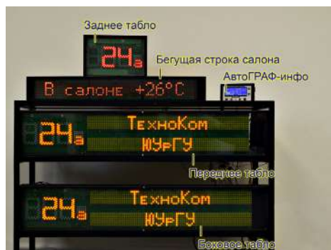
Рис.29. Внешний вид табло фирмы «Трансдеталь» (г. Н.Новгород).
