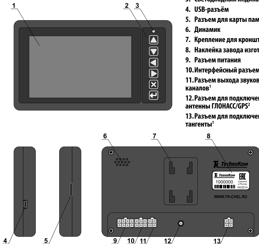
Рис.2. Составные части.
