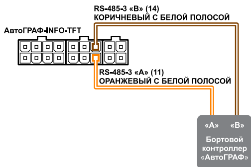
Рис.40. Схема подключения к контроллеру АвтоГРАФ.
