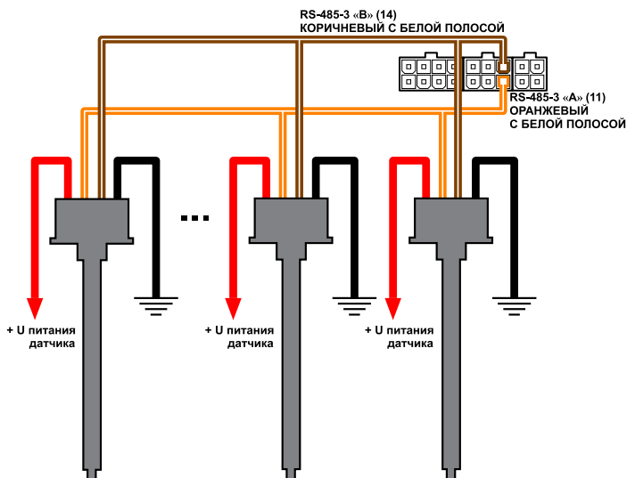
Рис.41. Схема подключения датчиков уровня топлива к дисплею.
