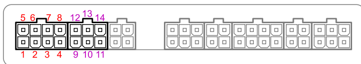
Рис.5. Интерфейсные разъемы дисплея «АвтоГРАФ-ИНФО» (5" TFT / microSD).
