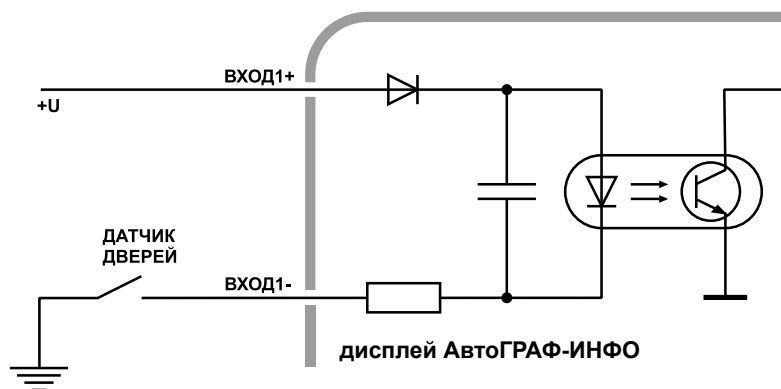
Рис.10. Подключение дискретного входы 1. Вариант 2.
