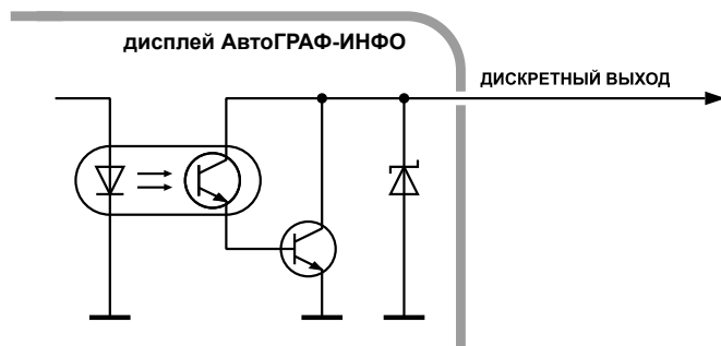
Рис.13. Подключение дискретного выхода.
