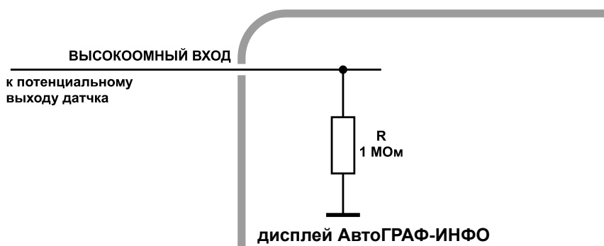
Рис.12. Подключение высокоомного входа.
