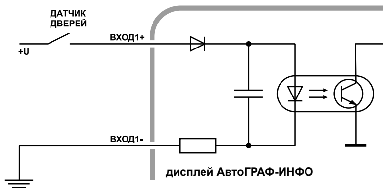
Рис.9. Подключение дискретного входы 1. Вариант 1.
