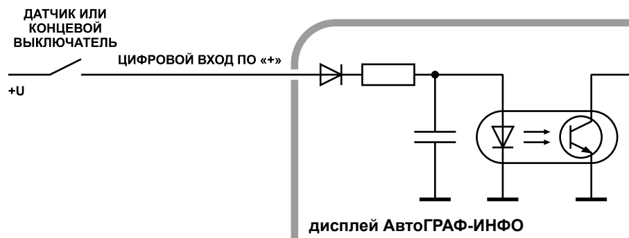
Рис.11. Подключение дискретных входов 2 и 3.
