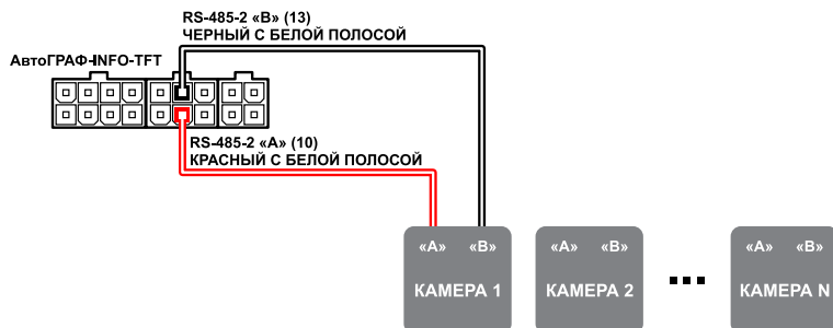
Рис.34. Схема подключения фотокамер.
