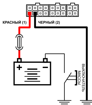
Рис.8. Подключение питания после выключателя массы.
