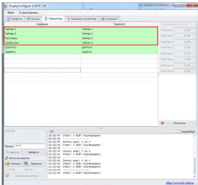
Рис.95. Вывод таймеров на рабочий экран.
